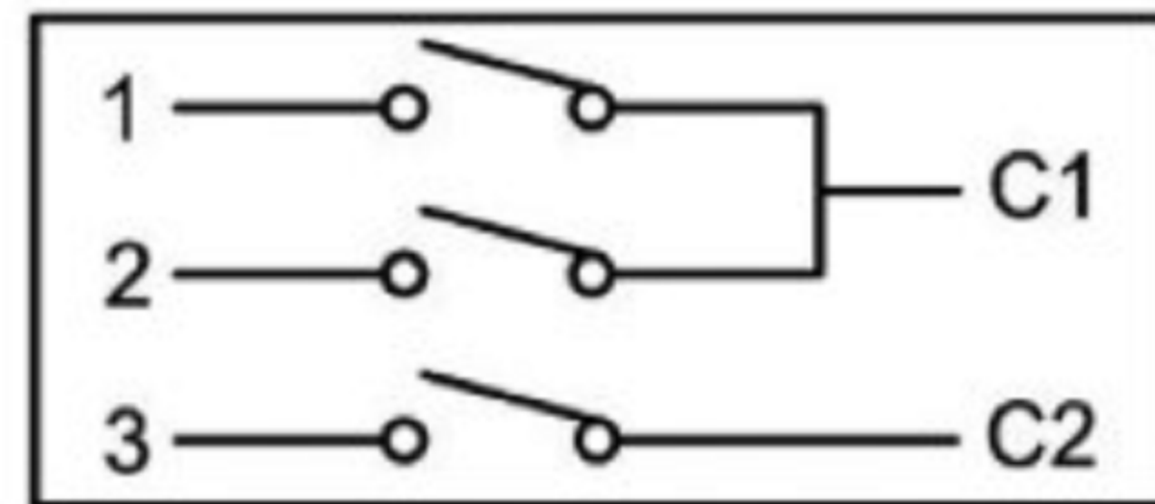
线路图 CIRCUIT DIAGRAM
