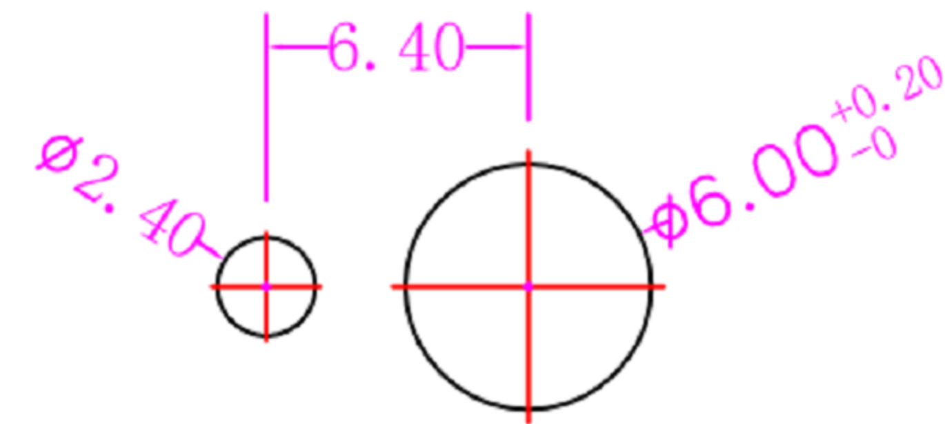
安装孔尺寸
