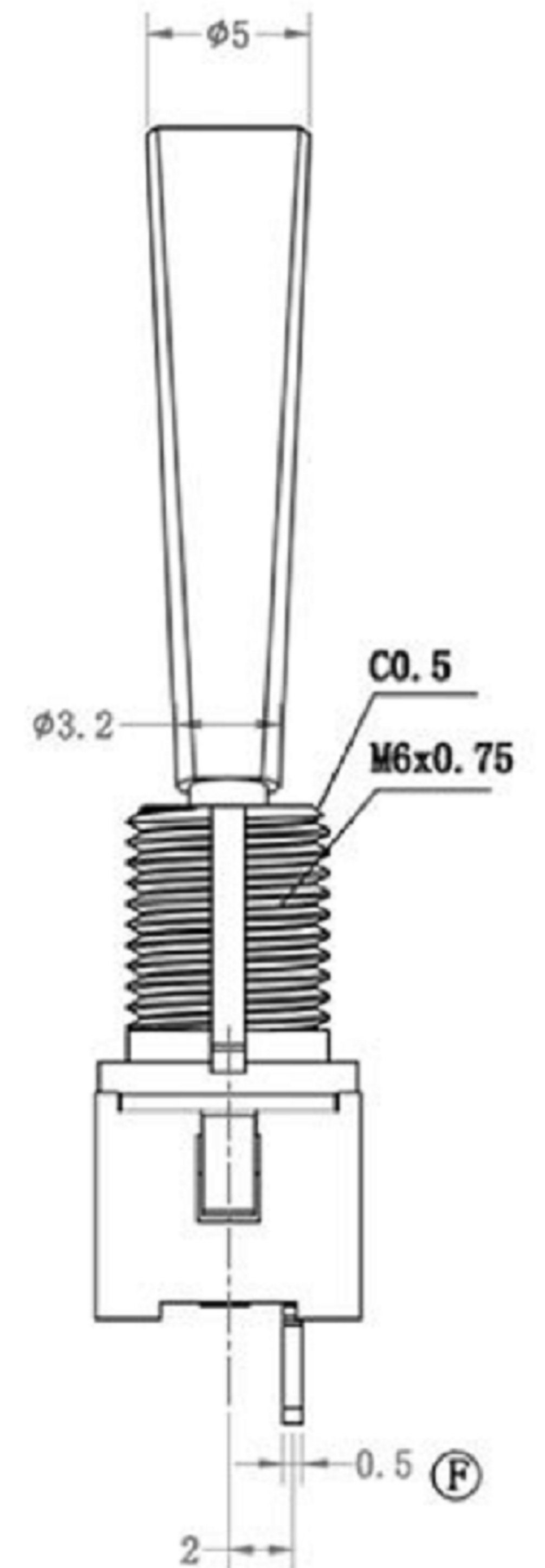
标注 A - F 为重点尺寸
