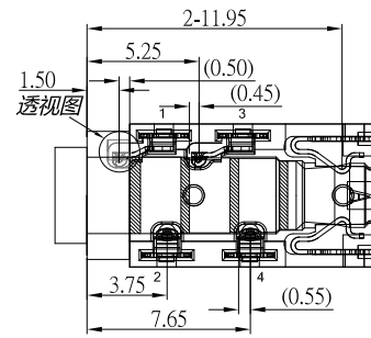
5 级插头接触点位置尺寸
