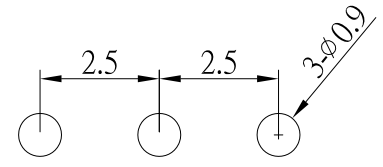
P.C.B LAND PATTERN
