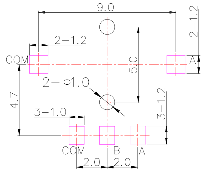
P.C.B LAYOUT
