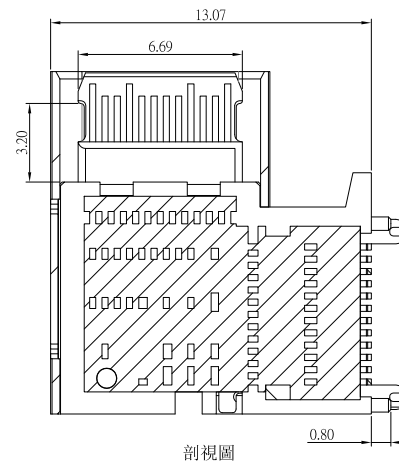
剖視圖
