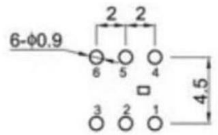
印制电路板 printed-circuit board
