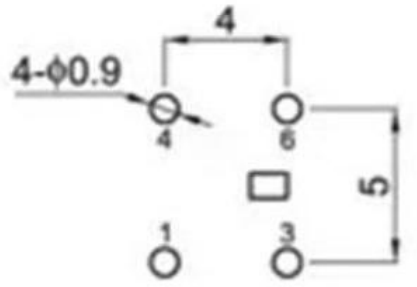
印制电路板 printed-circuit board
