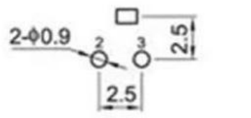
印制电路板 printed-circuit board
