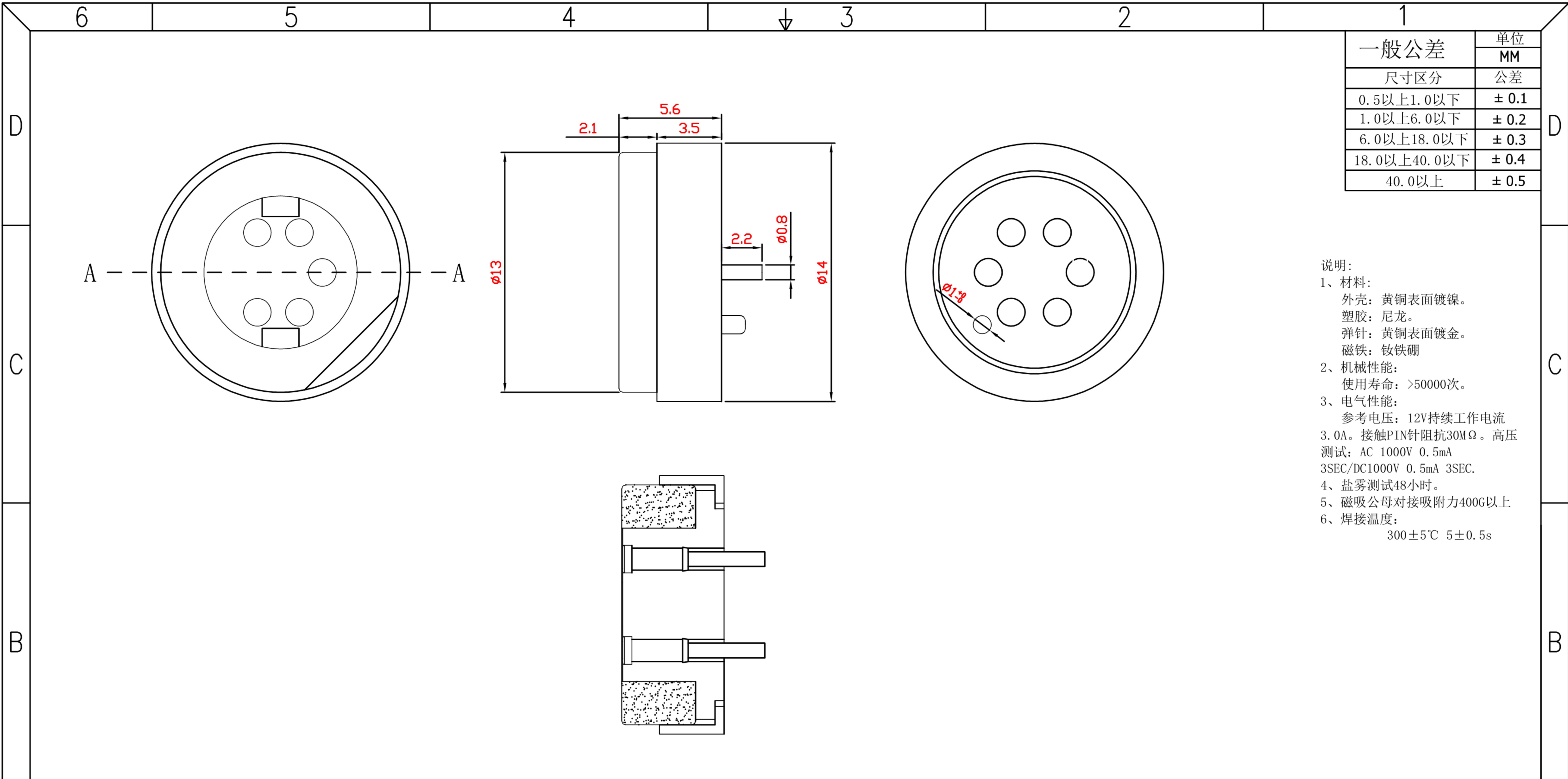
A-A剖
