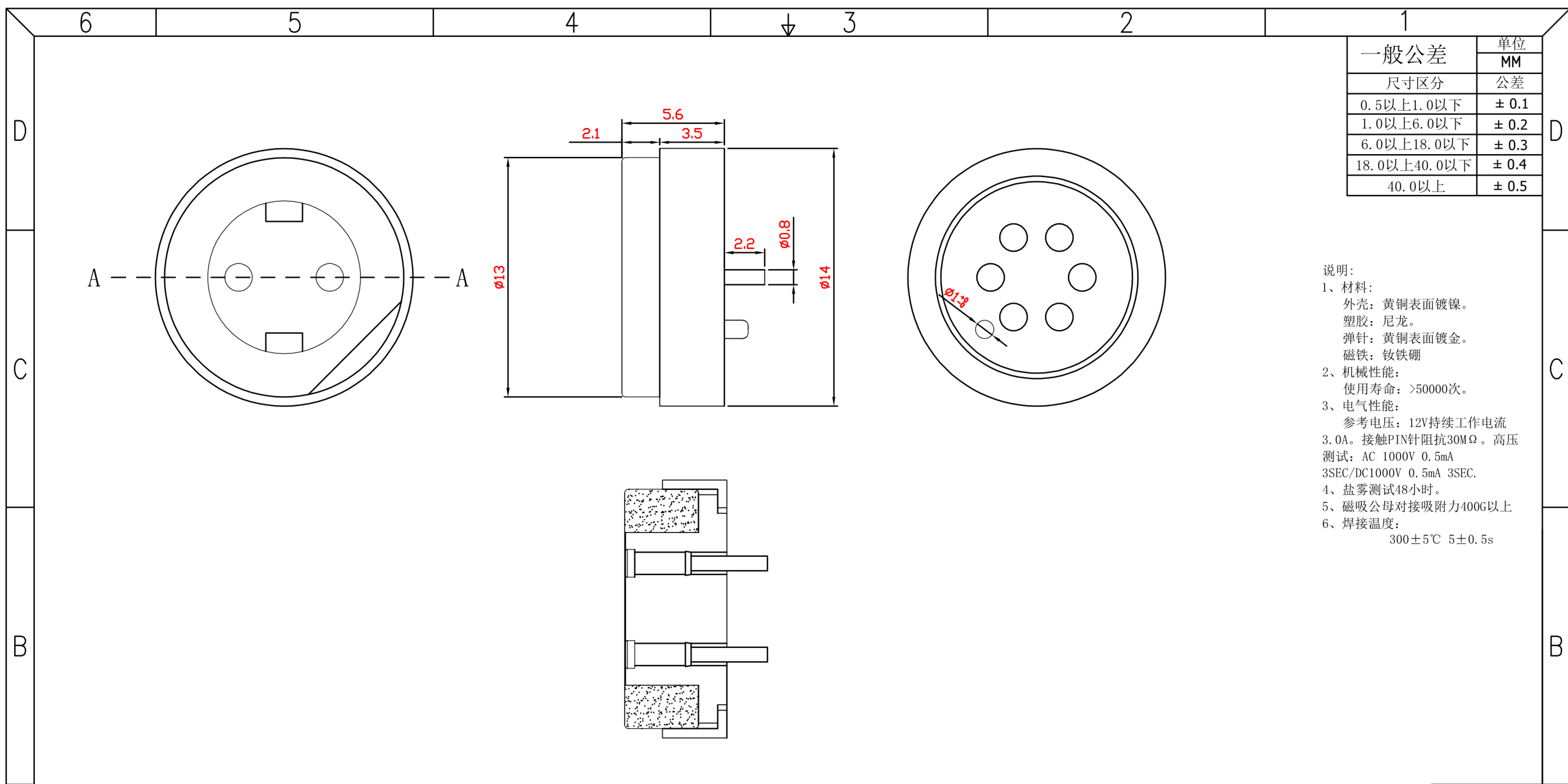
A-A剖
