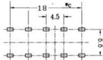
P.B.C LAYOUT
