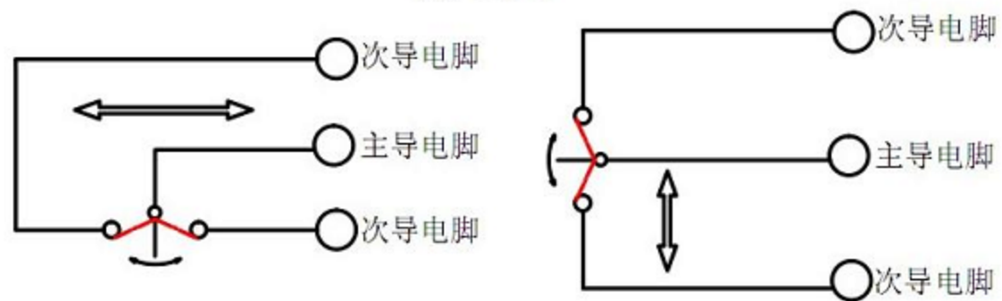
原理图
