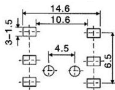
P.C.B. Pattern
