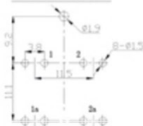
印制板开孔尺寸(±0.1mm)
