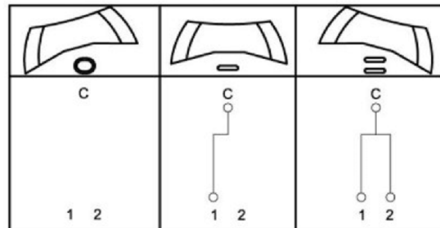
线路/ Circuit
