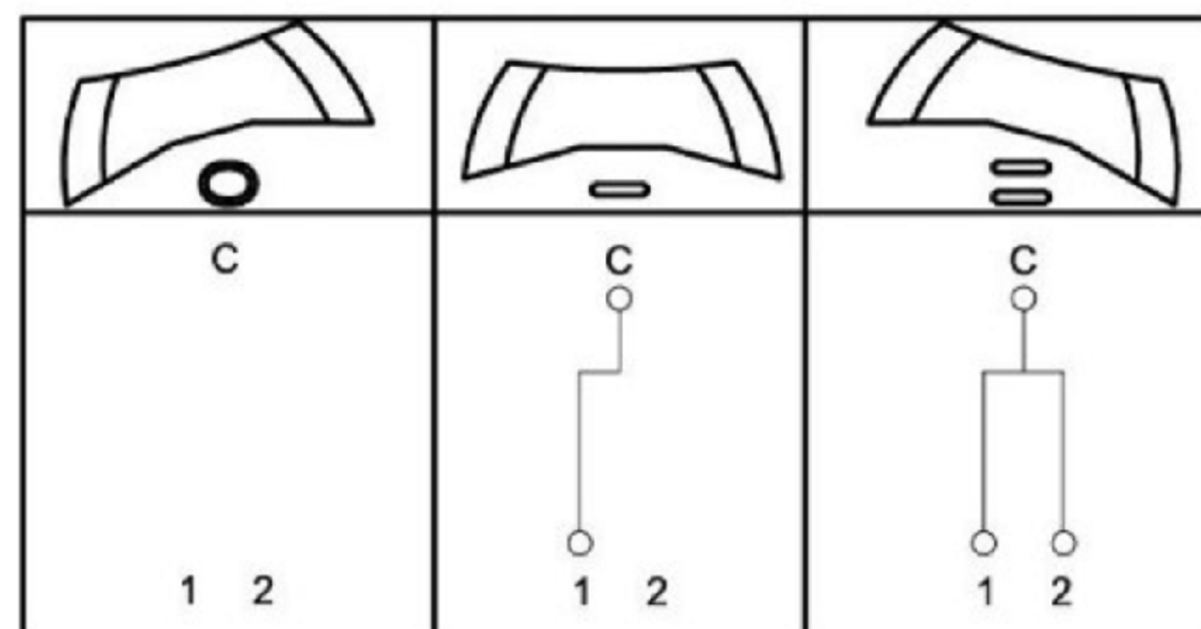
线路/ Circuit
