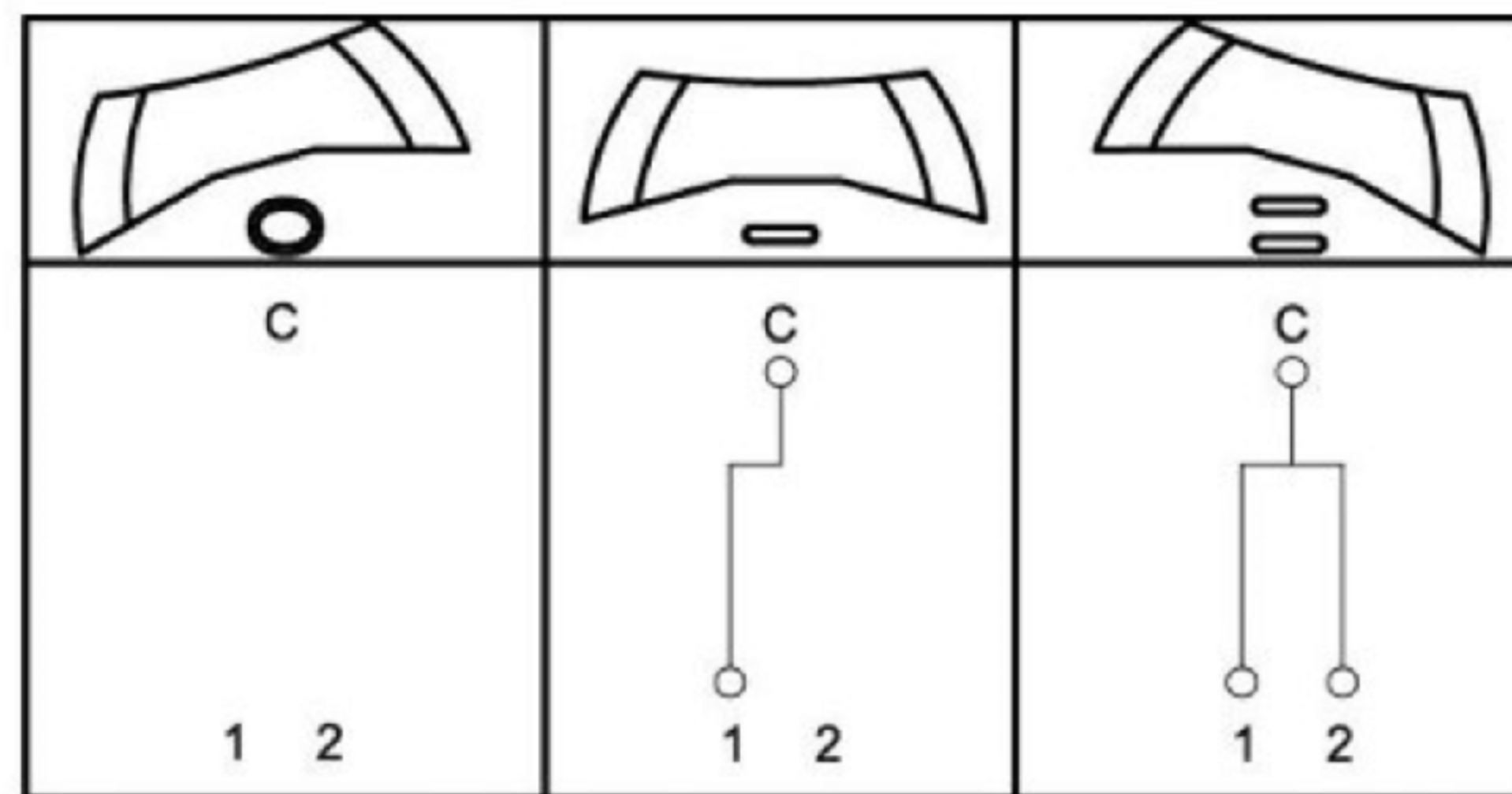
线路/ Circuit
