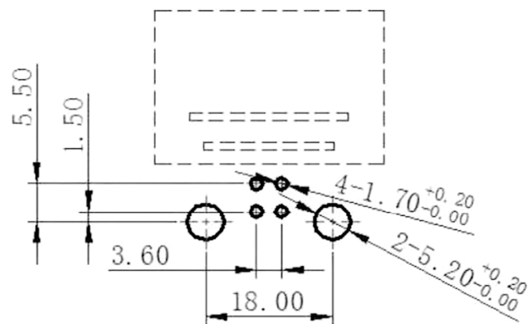
推荐 PCB 开孔尺寸
