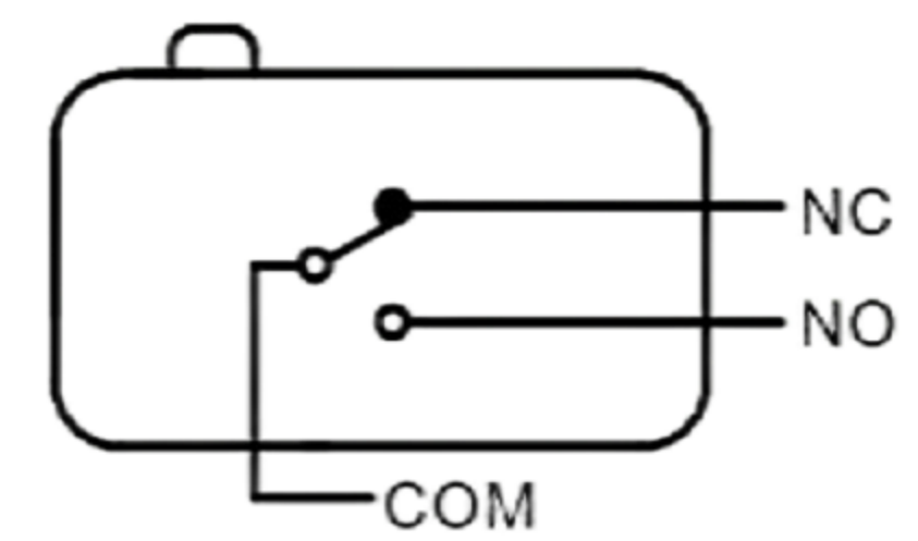
转换型SPDT
