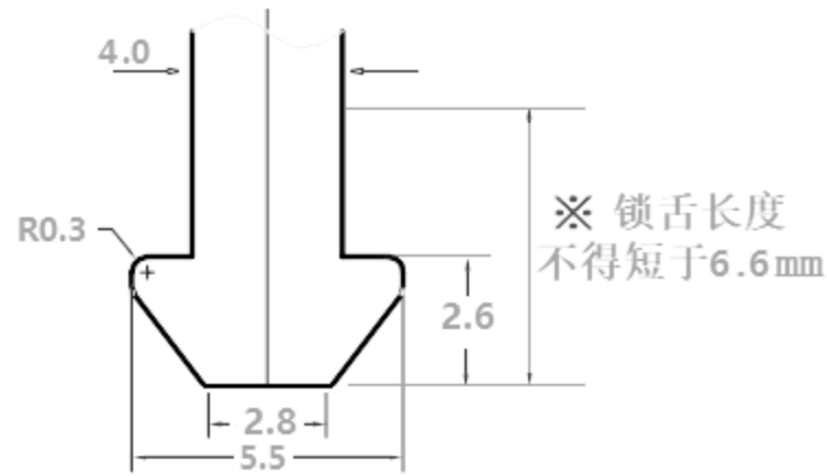
锁舌参考尺寸
