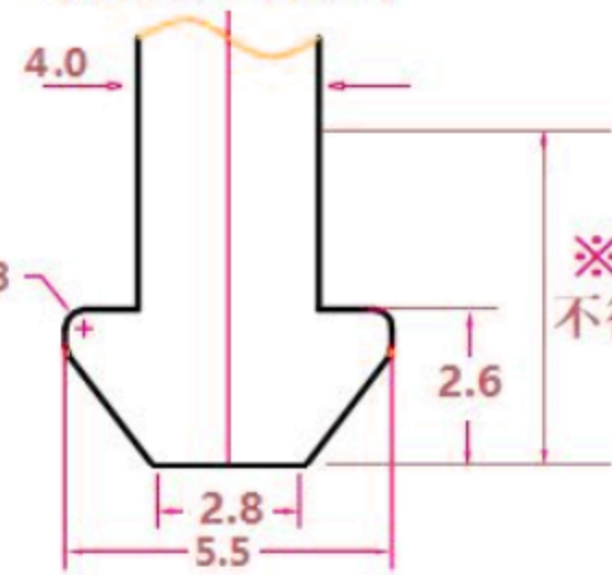
锁舌参考尺寸
